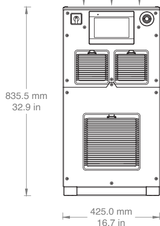
VISTA FRONTALE
