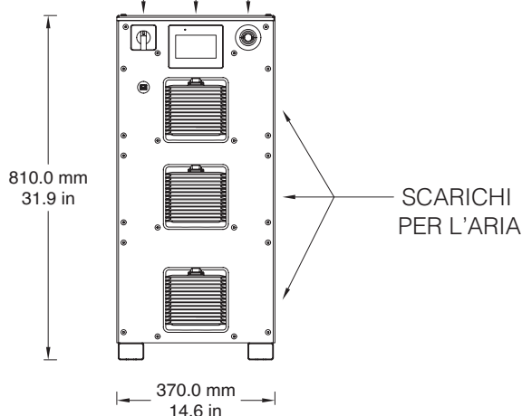
VISTA FRONTALE
