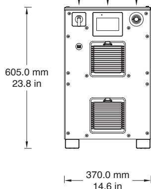
VISTA FRONTALE
